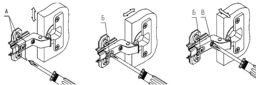
Схема 5. Регулирование положения фасада
