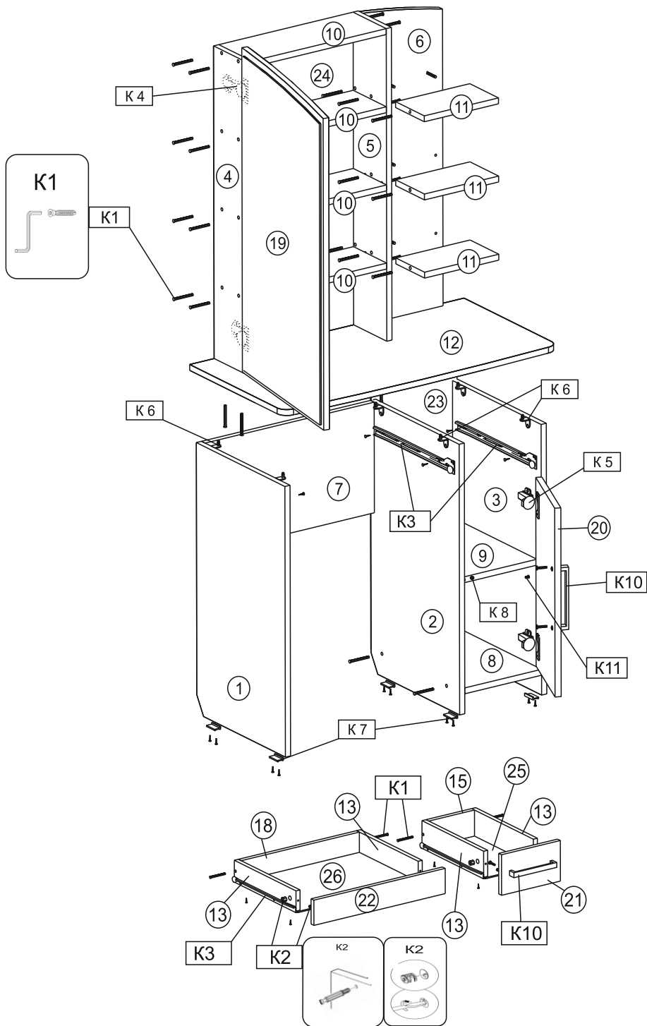
Схема 1: Корпус трюмо
